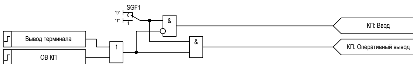
Рисунок 2.29 – Функциональная схема управления режимами работы контроллера присоединения
