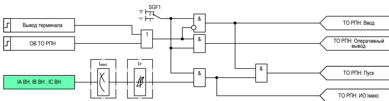
Рисунок 2.10 – Функциональная схема логики ТО РПН
