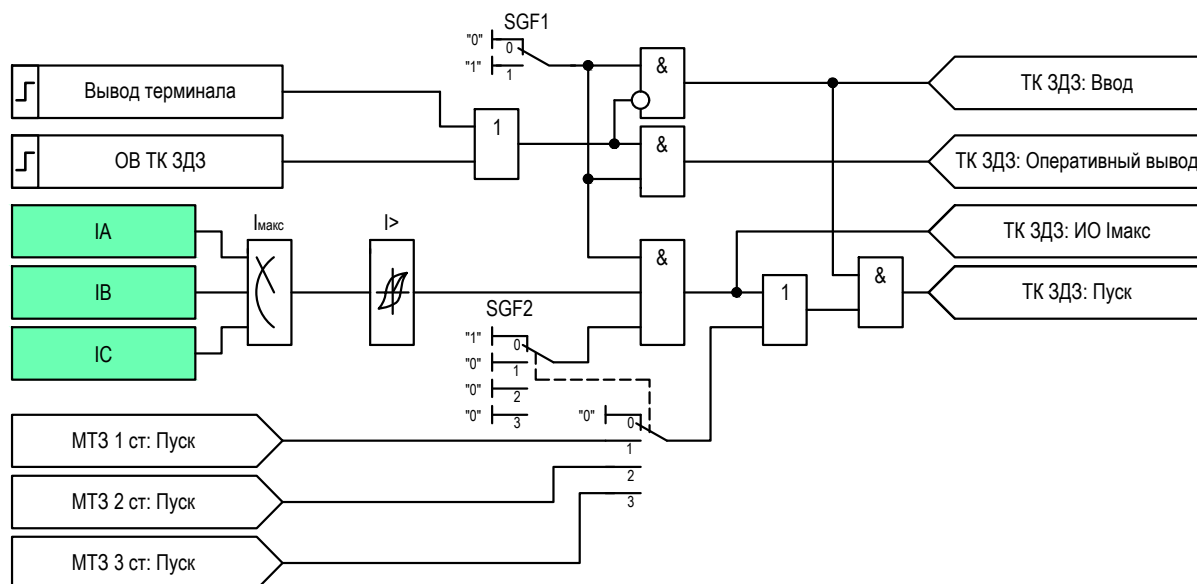
Рисунок 2.9 – Функциональная схема логики ТК 3Д3
